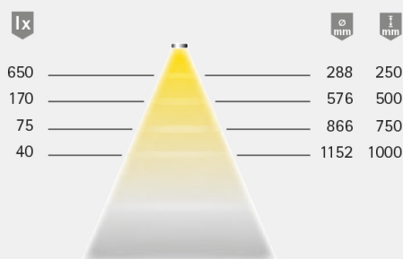
Diagrama de distribución luminosa / 60° (por módulo de luz)
